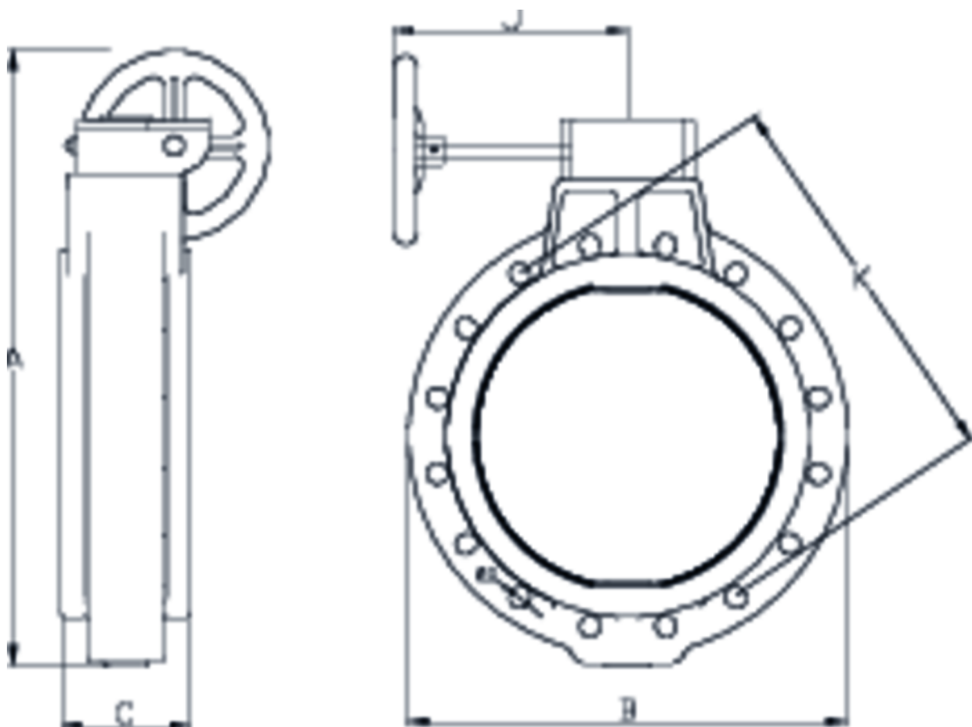
ITEM 187XXL | Vanne papillon Implex à brides avec réducteur manuel Ø400
