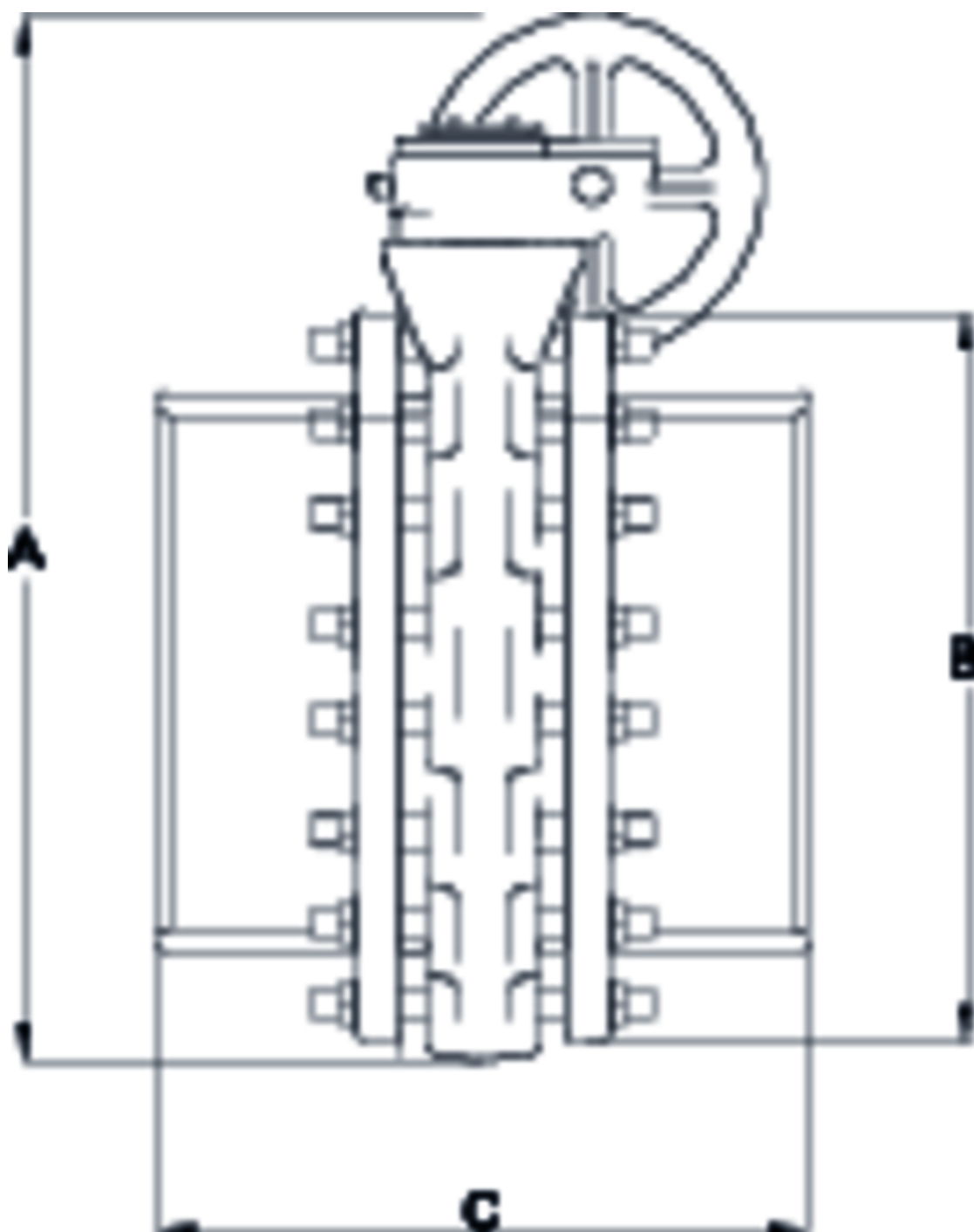
ITEM 185XXL | Válvula de mariposa Implex manoreductor Ø400
